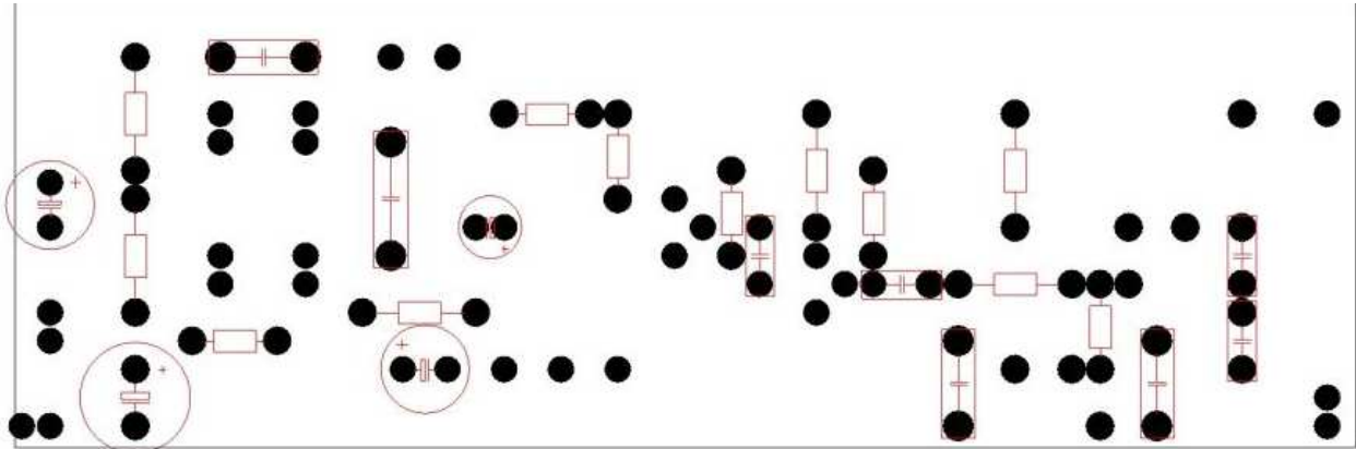
Печатная плата со стороны монтажа
