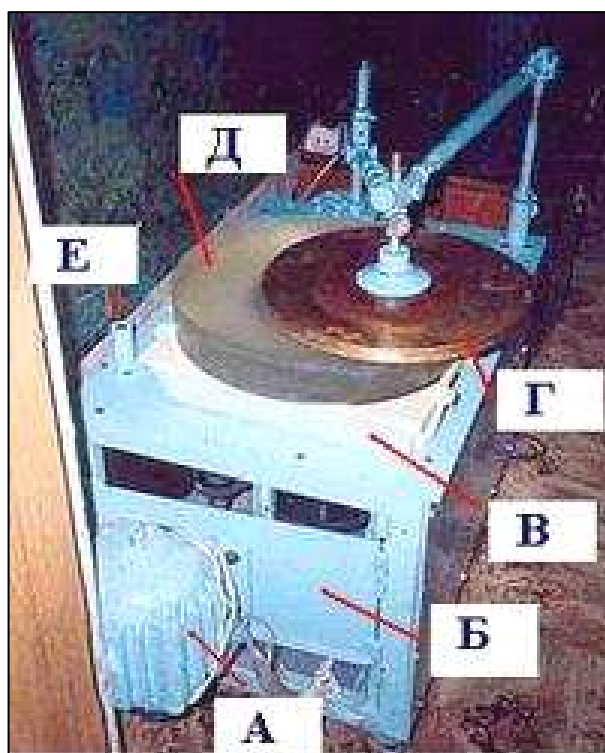
По бокам станок прикрывался листами из текстолита, Рис.2
